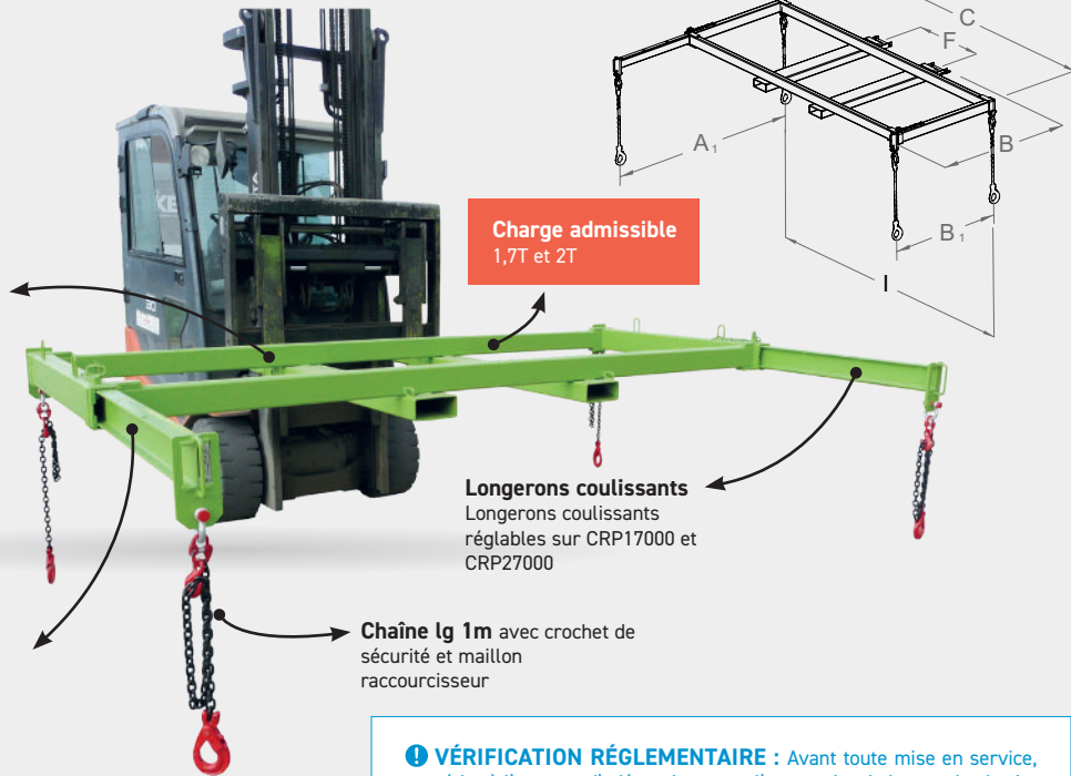
CRP17000 Blocage sur fourches par axes amovibles
