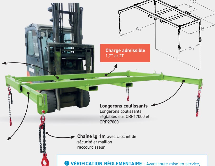
CRP17000 Blocage sur fourches par axes amovibles
