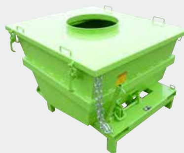
Couvercle amovible
