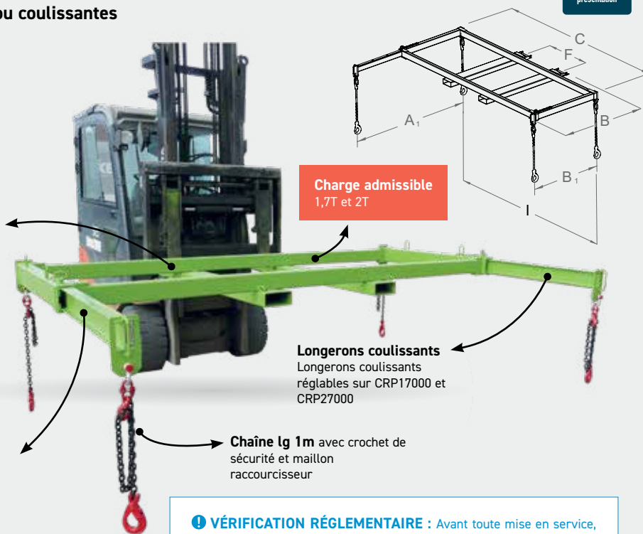
CRP17000 Blocage sur fourches par axes amovibles
